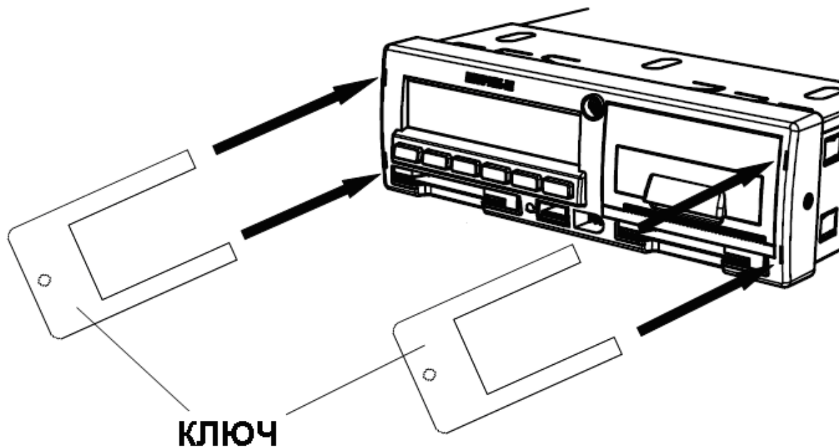
Рисунок 4 – Извлечение тахографа
