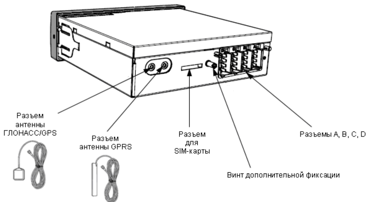
Рисунок 3 – Внешний вид задней панели тахографа
