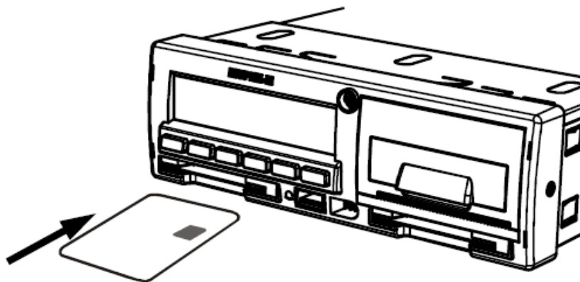
Рисунок 5 – Вставка карты водителя в картоприемник основного водителя «1»
